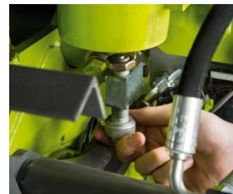
Ayuda de ajuste para el reajuste de la piedra de afilado
