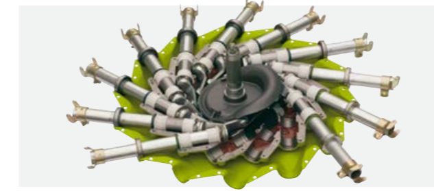
Fiabilidad sin mantenimiento: El corazón del LINER es el plato excéntrico en baño de aceite.
